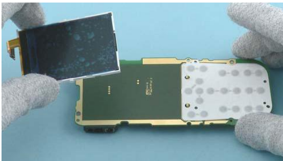
23) Remove the LCD.
