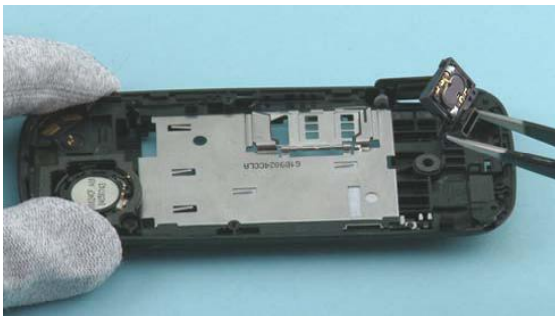
17) Remove the EARPIECE MODULE using tweezers.
